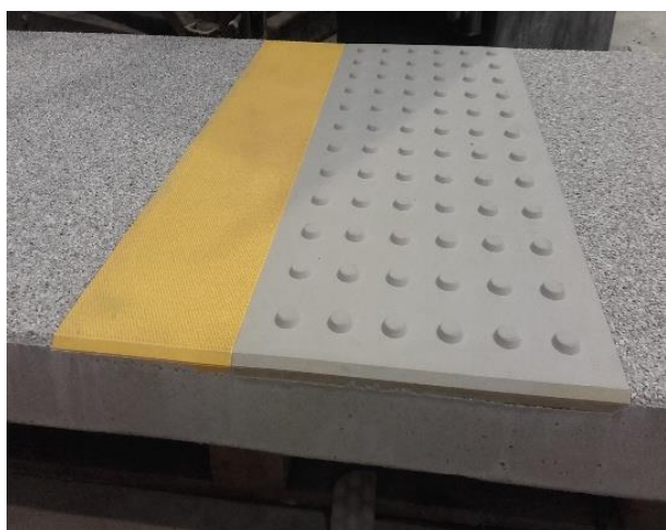
Rysunek 4.3: Sienkiewicz MAT-BUD Sp. z o. o. – płyta peronowa z odkrytym kruszywem – wariant podstawowy
