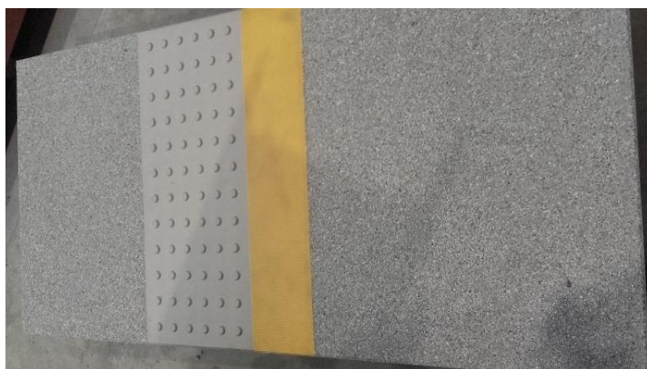
Rysunek 4.3: Sienkiewicz MAT-BUD Sp. z o. o. – płyta peronowa z odkrytym kruszywem – wariant podstawowy
