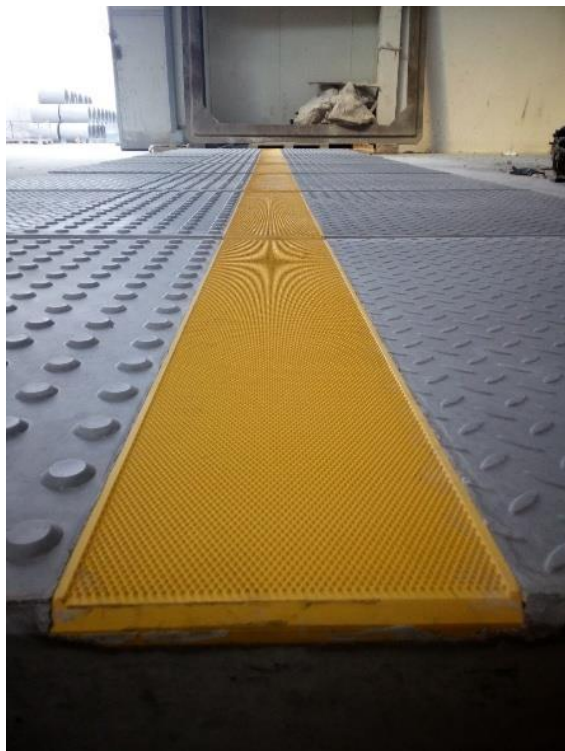
Rysunek 4.2: Sienkiewicz MAT-BUD Sp. z o. o. – płyta peronowa klasyczna betonowa – wariant podstawowy
